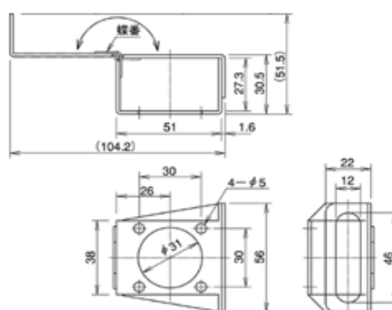
SPT-L3
