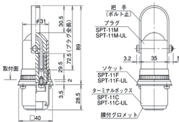
SPT-11 1回路
