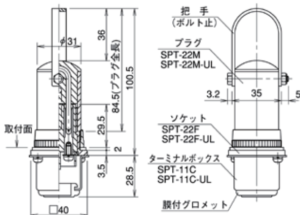
SPT-22 2回路
