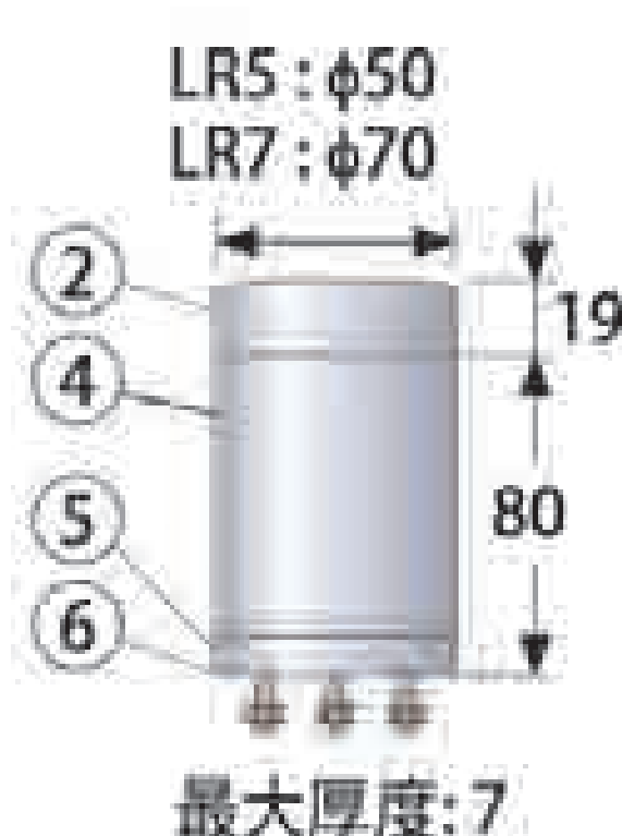
安裝 A [WT]直接安裝 / 電纜 接線端子 (主體元件)
