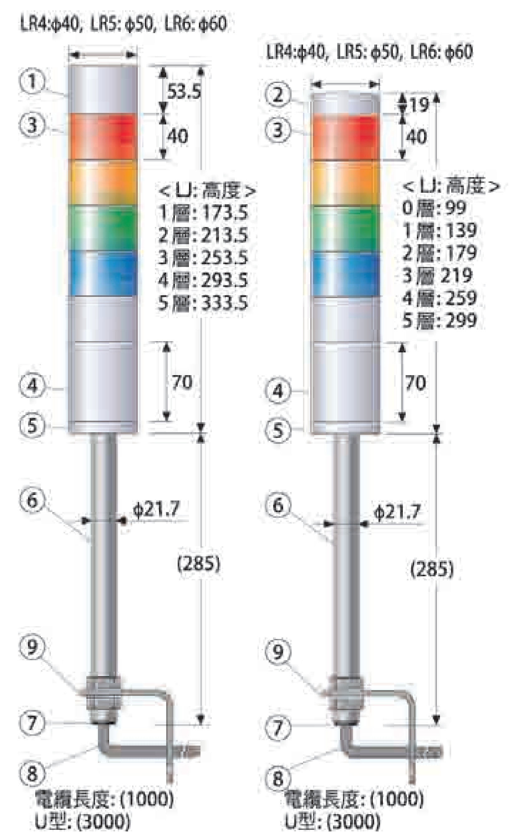
安裝 B [LJ] 桿式安裝，含 L 型支架 和電纜 (02：直流24V)
