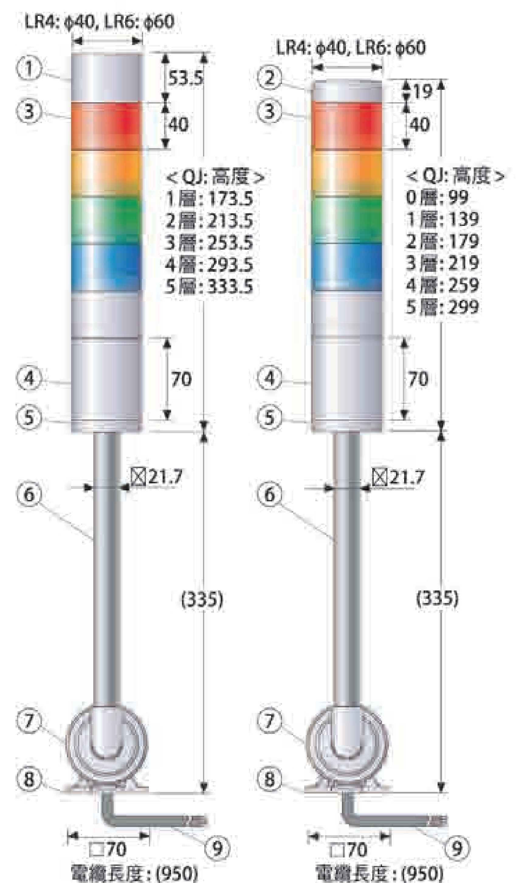
安裝 C [QJ] 桿式安裝，含折彎底座和電纜 (02：直流24V)
