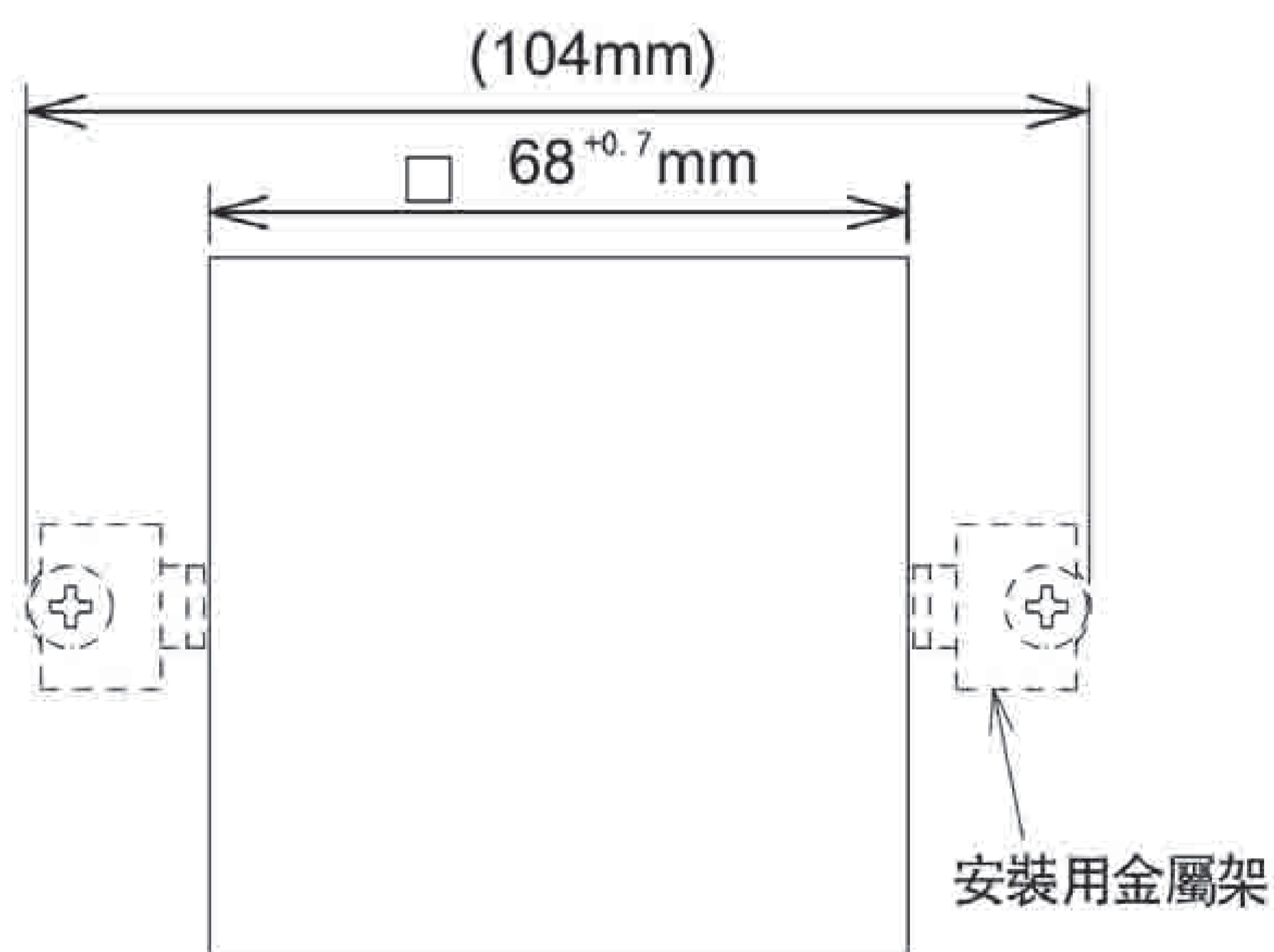
背面安裝尺寸圖
