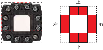
端子配置位置図 (端子部背面側から見る)
